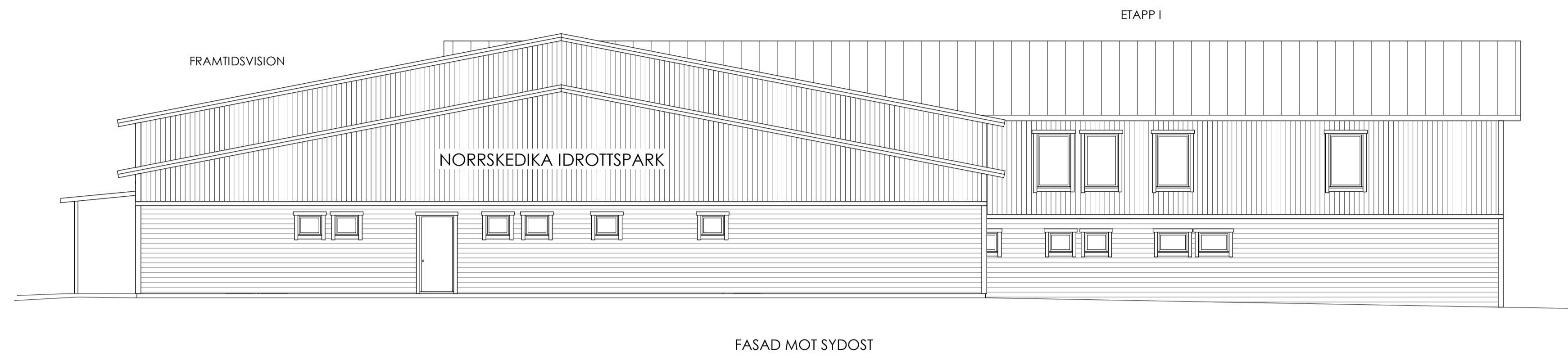
FASAD MOT SYDOST
